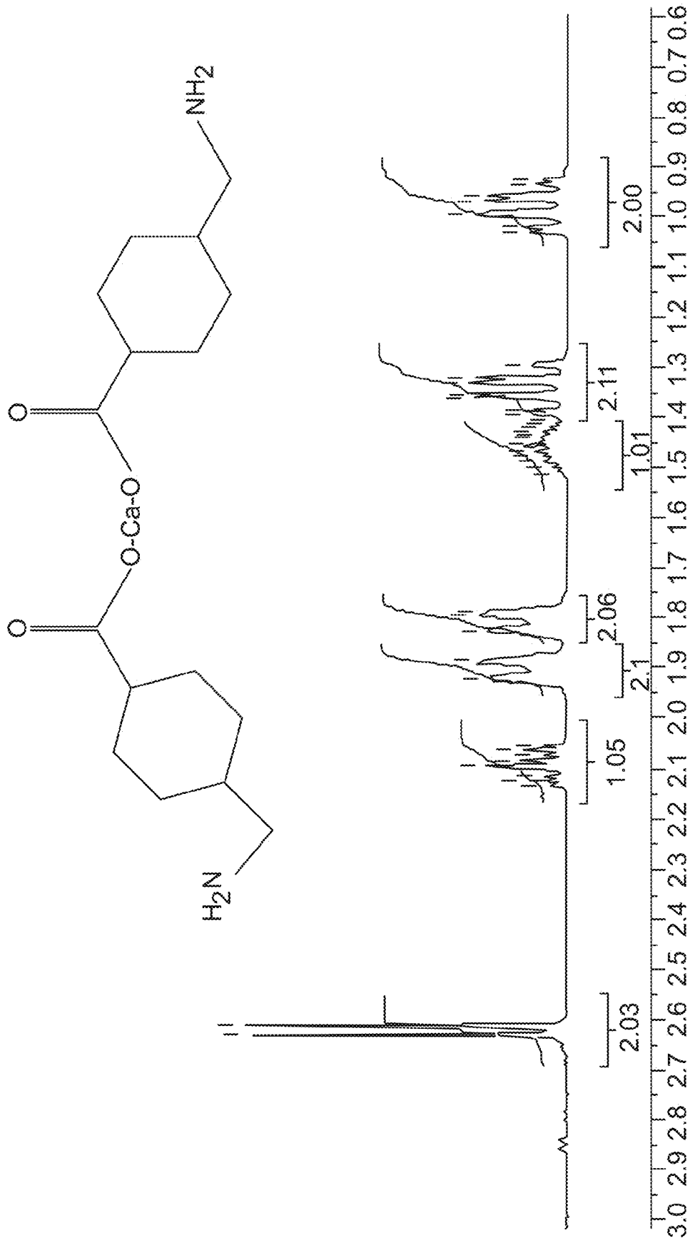
Calcium bis tranexamate in D 2 O
